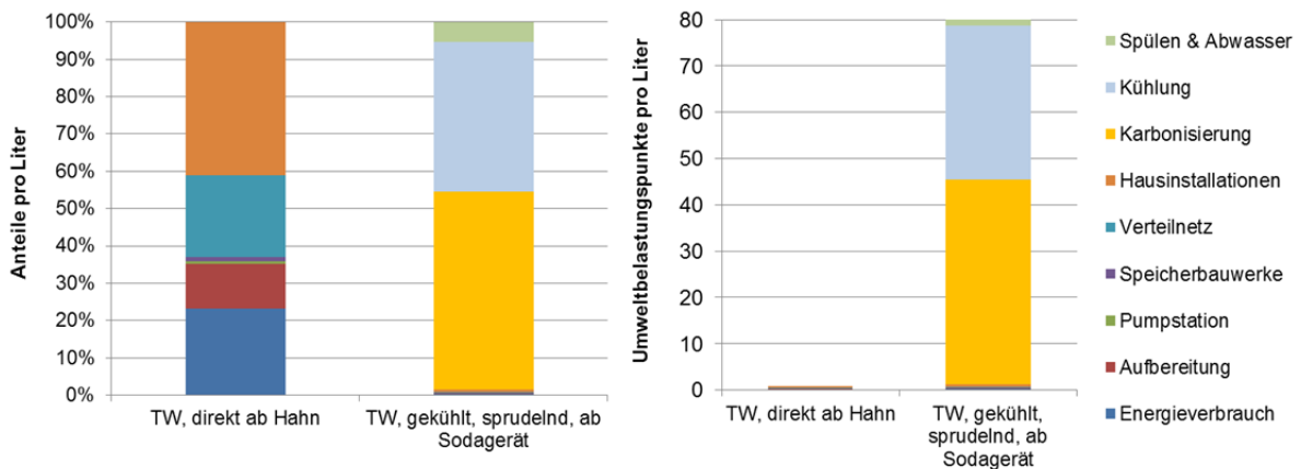
Fig.2 Prozessanteile an der Gesamtumweltbelastung nach der Methode der ökologischen Knappheit (2013) für Trinkwasser
