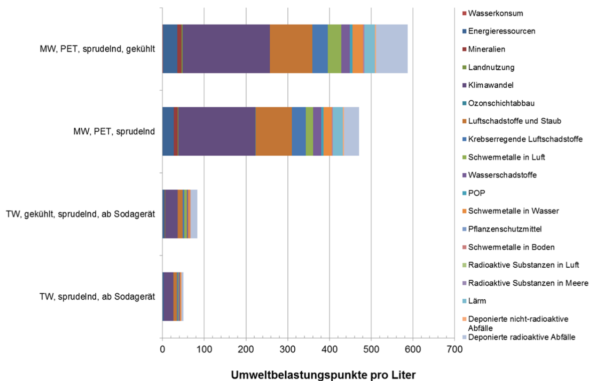
Fig. 3 Vergleich der verschiedenen Varianten für kohlenensäurehaltiges Wasser mit der Methode der ökologischen Knappheit 2013
